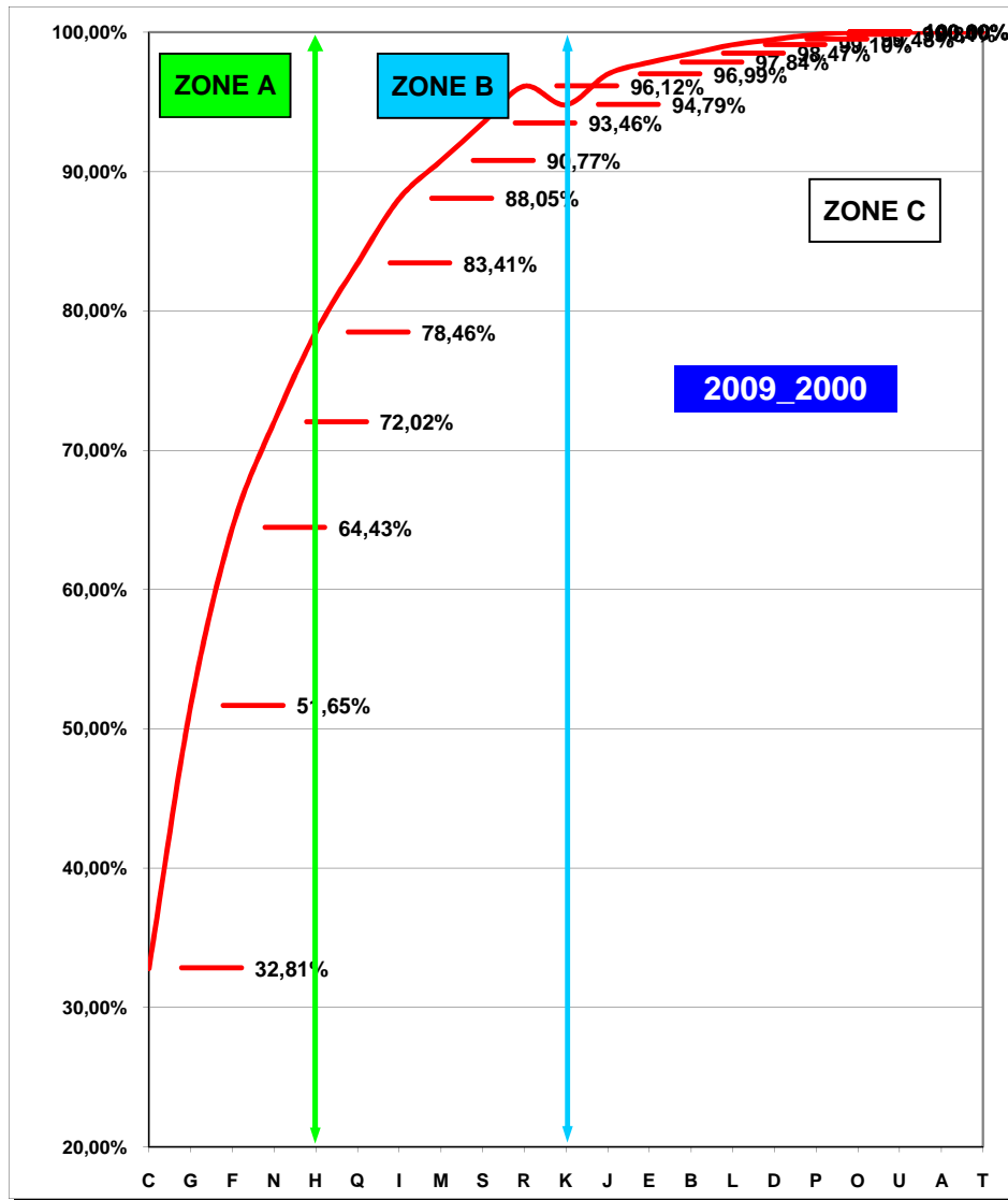
G12 - Emplois cumulés par secteur en pourcentage Analyse des 80/20 - Diagramme de Pareto 2009 PROVISoire
